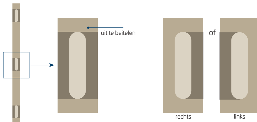
PORTIXX RF30 OMKEERBAAR SCHARNIER
