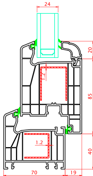
A-A' SECTION
